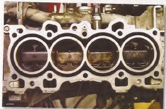
Motor policilíndrico
